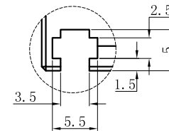
视图A 比例2:1
