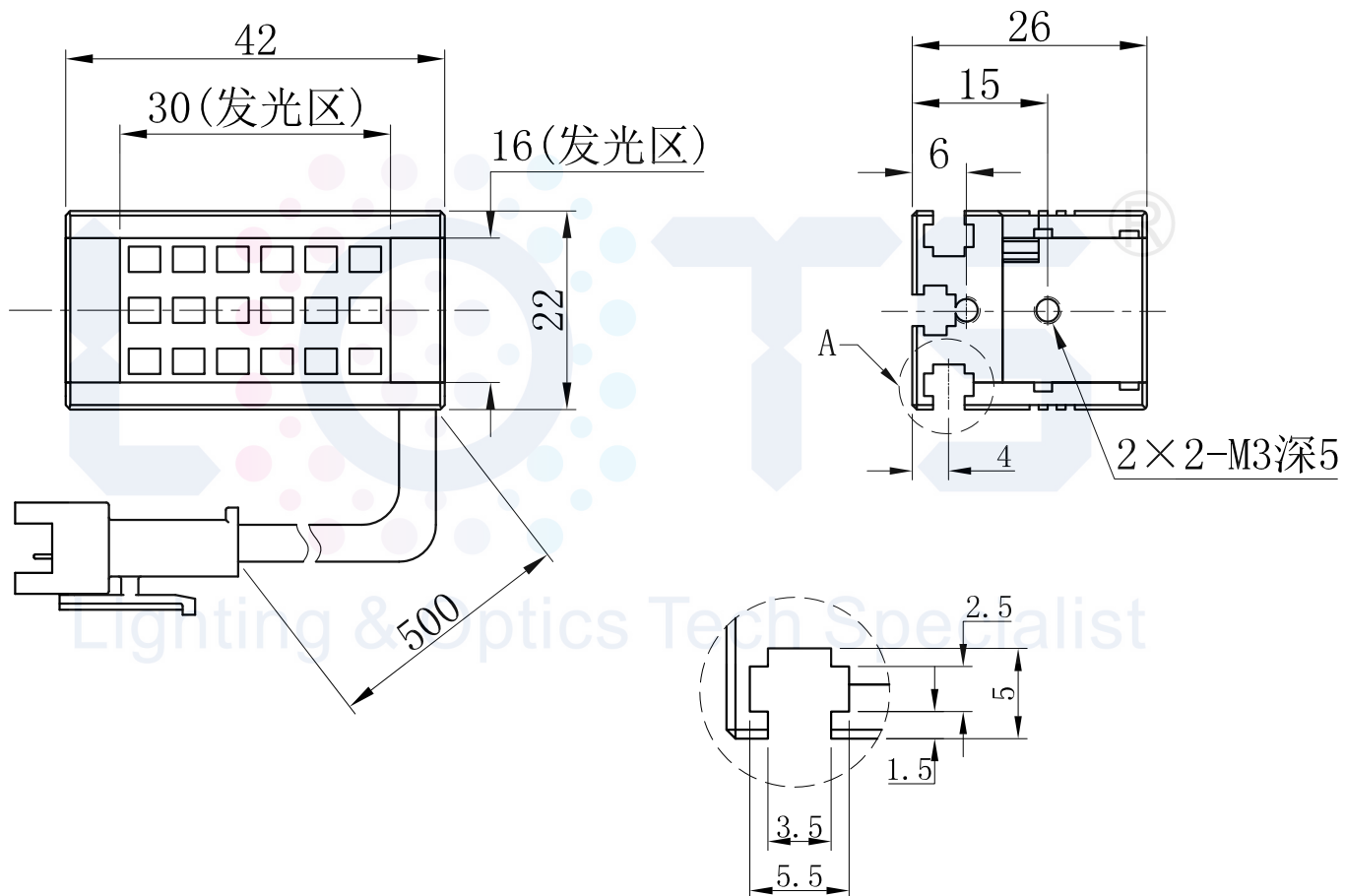
视图A 比例2:1
