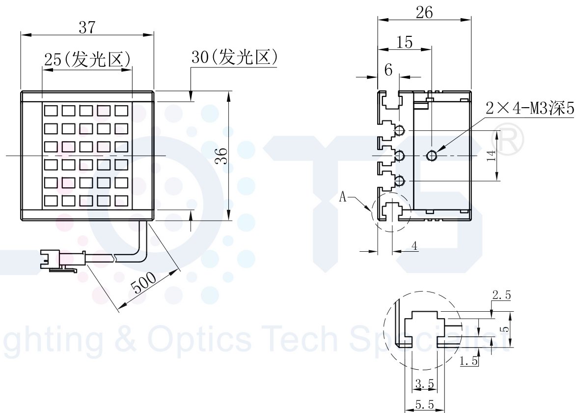
视图A 比例2: 1
