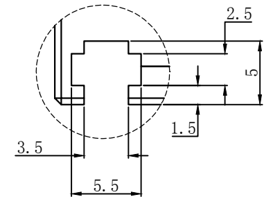
视图A 比例2:1
