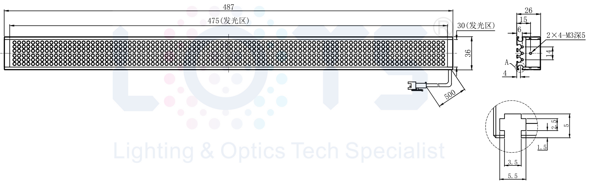
视图A
