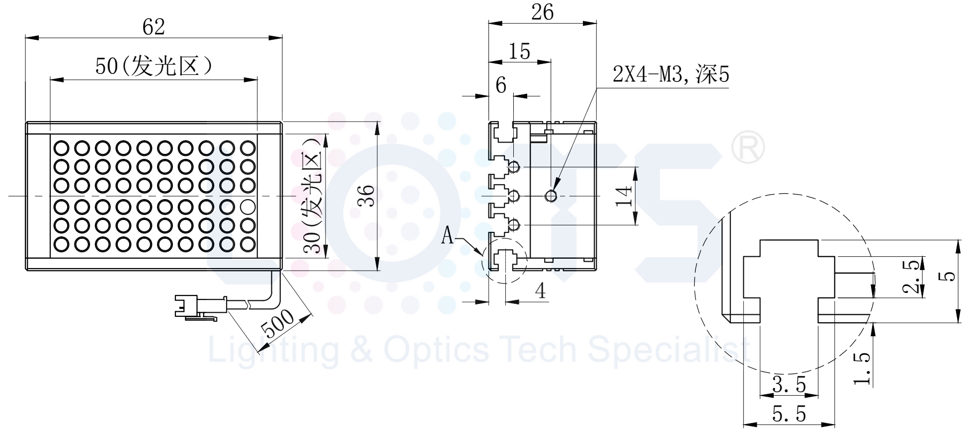
视图A 比例4: 1
