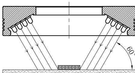
照明示意图
