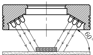
照明示意图
