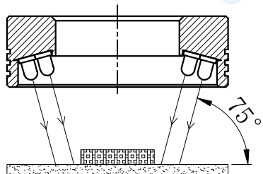
照明示意图
