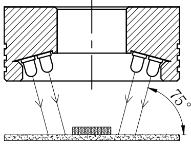
照明示意图
