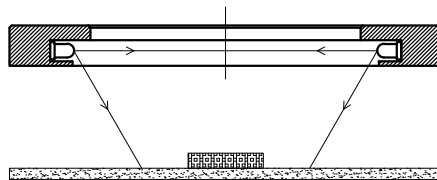
照明示意图
